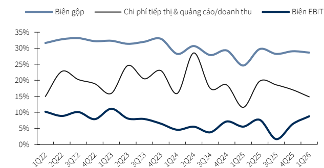
Biểu đồ 25. Biên lợi nhuận hoạt động EBIT (không bao gồm tài
